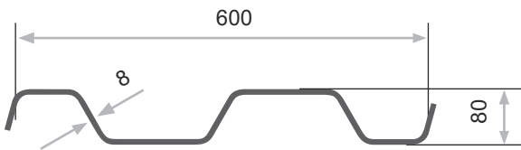
Profil KD 6/8
